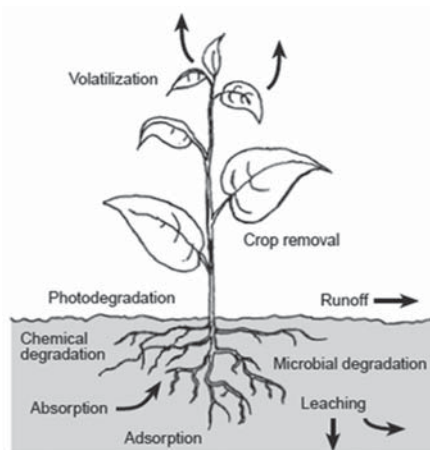
圖 1.除草劑施用後在環境中吸附、轉移及分解過程。(Fishel, 2010)
