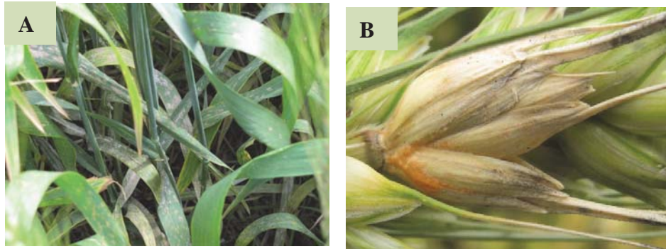
圖八、小麥罹病病徵。A：白粉病。B：赤黴病。
